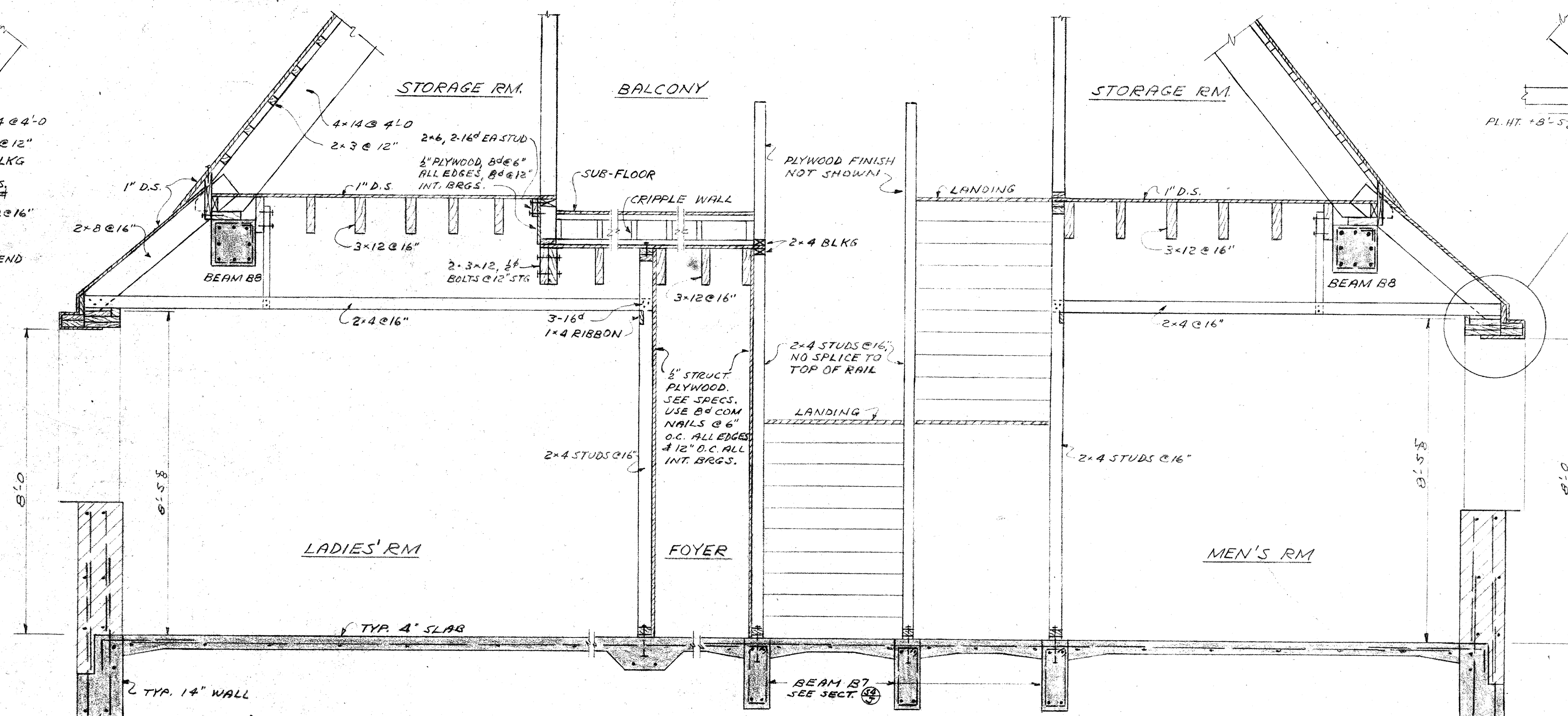
SECTION B SCALE: 3/8"=1'-0"
